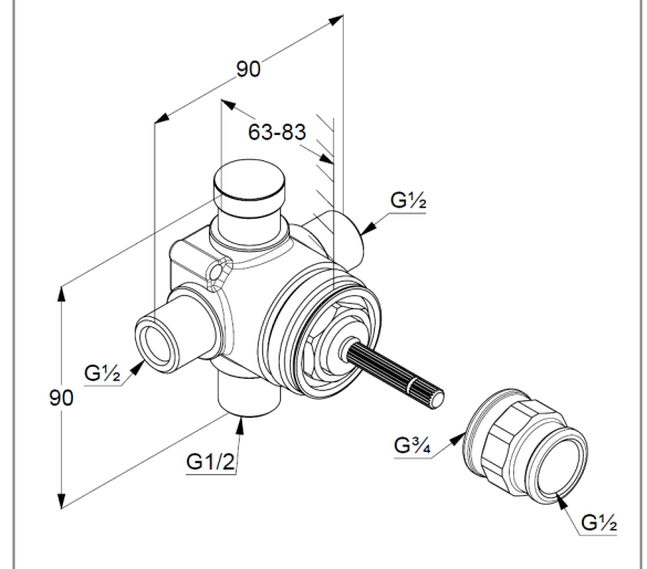
Maßzeichnung
