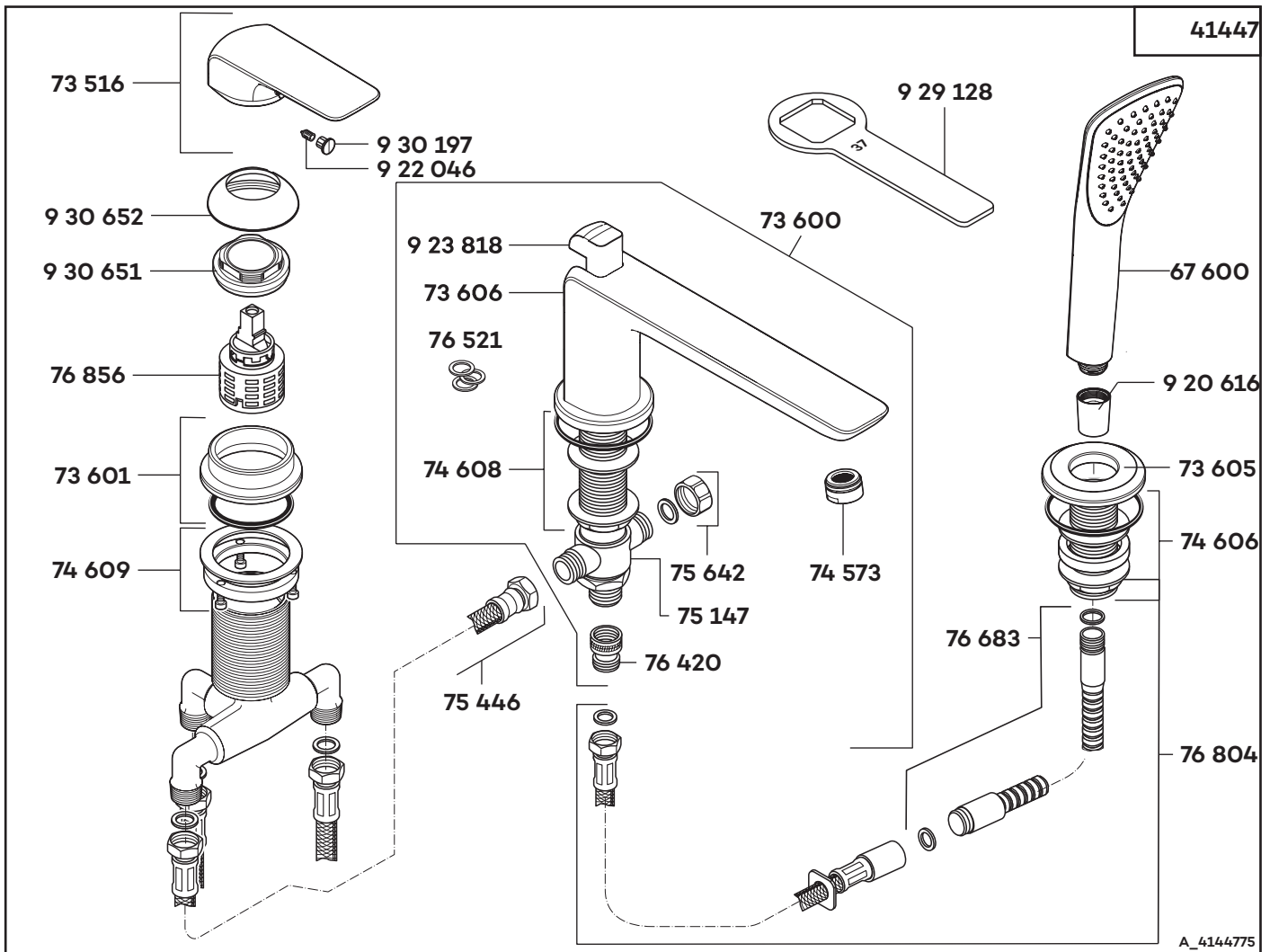
41447 Wannenfüll- und Brause-Einhandmischer DN 15 single lever bath- and shower mixer DN 15 ééngreeps bad-/douchemengkraan 1/2"
